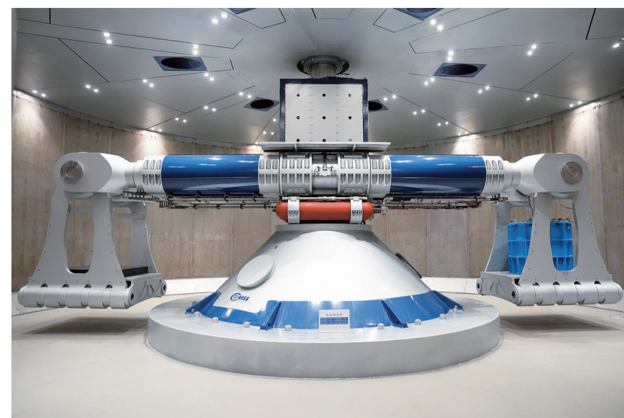
9月29日拍摄的超重力离心模拟与实验装置启动的首台离心机主机“CHIEF1300”。
