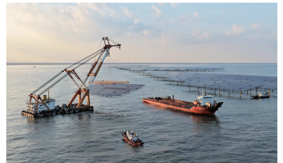
12月24日,工人在位于河北省昌黎县海域的海上光伏电站试点项目建设工地操作机械作业(无人机照片)。近日,中国华电集团有限公司河北分公司在河北省昌黎县海域投资建设的河北省海上光伏电站试点项目,正在按照节点要求扎实推进。据介绍,该项目装机容量465.6兆瓦,建成并网投运后,将为推动海洋经济高质量发展,落实“双碳”目标注入强劲动能。【新华社记者 杨世尧 摄】
