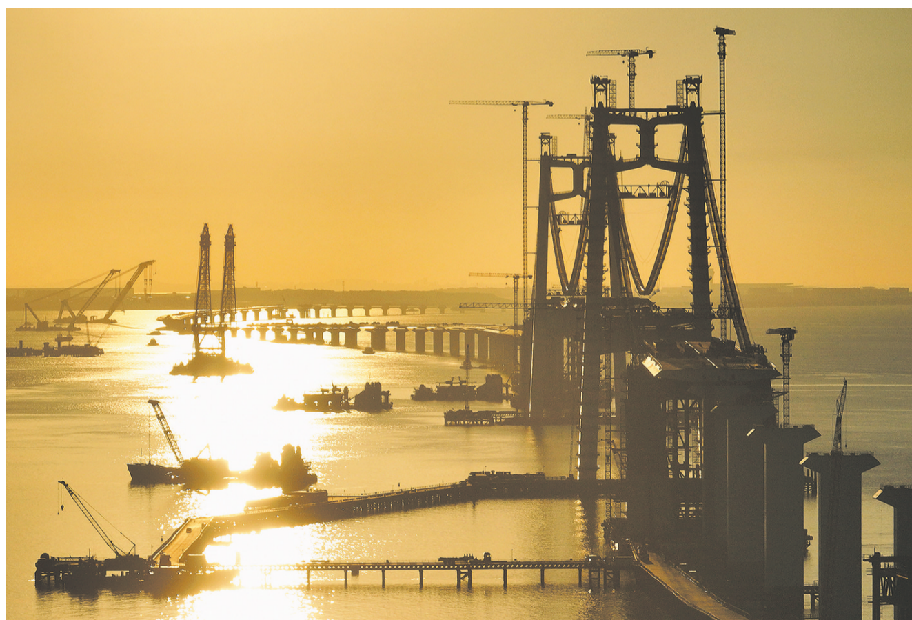
7月8日拍摄的建设中的厦金大桥(厦门段)项目(无人机照片)。
