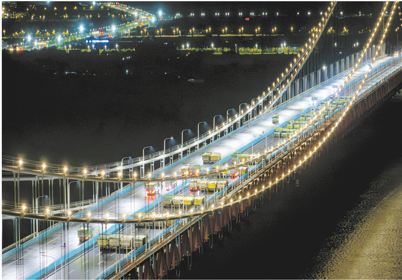
这是8月30日拍摄的燕矶长江大桥静态荷载试验现场(无人机照片)。 8月30日晚,由湖北交投集团投资建设的燕矶长江大桥正式进入荷载试验阶段。180台重型载重车在上下层桥面同步布设,开展为期5天的静态和动态荷载试验,全面检验大桥承载力和安全性,为后续项目建成通车提供科学依据。 燕矶长江大桥采用双塔单跨设计,主跨1860米一跨过江,上层为高速公路,下层为城市快速路,未来将成为鄂东空铁、空陆联运立体交通的重要过江通道,是推动黄冈、鄂州、黄石三市跨江联动、一体化发展的关键工程。 【新华社记者 肖艺九 摄】
